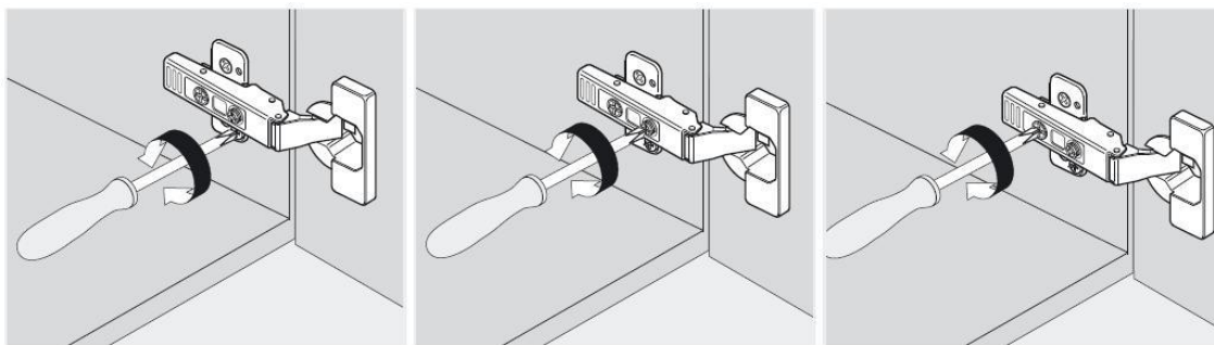
Ajuste altura
